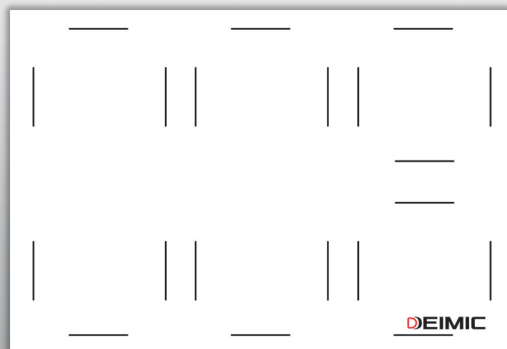
Włącznik czteropolowy Num. 28.TS4R2W
