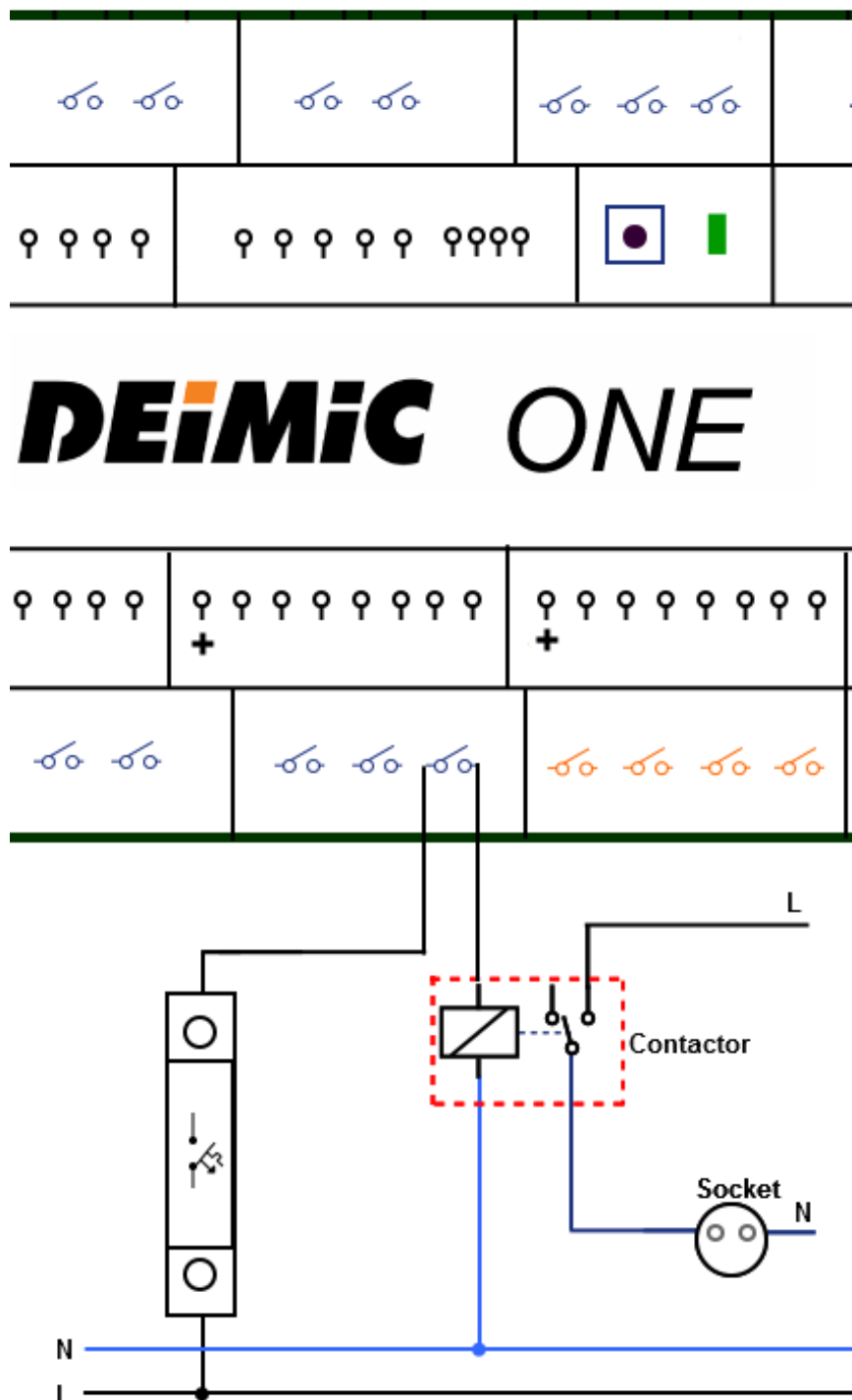
Ryc. 7. Schemat podłączenia wyjść (stycznik) do DEiMiC ONE EXPANDER .
