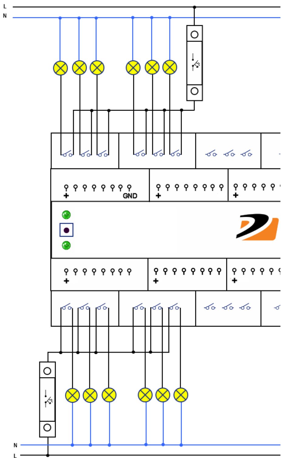
Ryc. 3. Schemat podłączenia wyjść (światła) do DEiMiC ONE EXPANDER .
